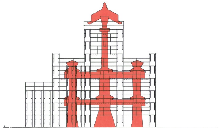
大鳥居外部足場図
